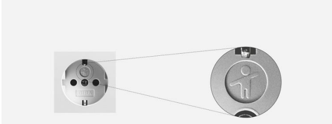
GIRA Steckdosen mit integriertem erhöhten Berührungsschutz
